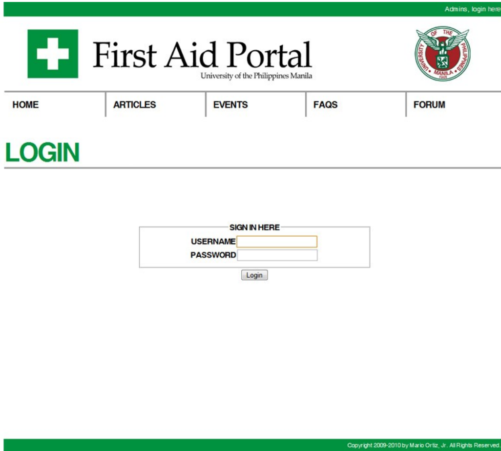
Fig. 38 Login Page
