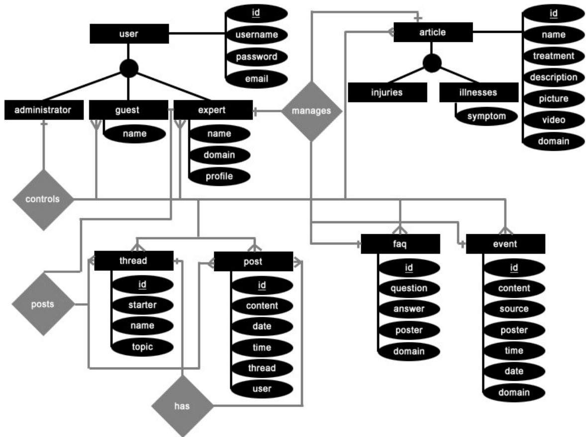
Fig. 1 The Entity-Relationship Diagram (ERD)
